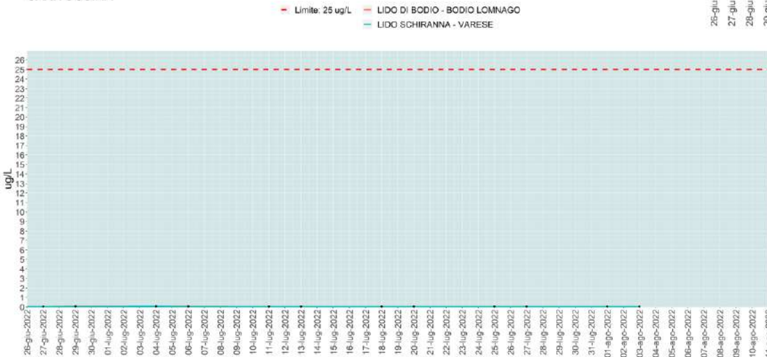
SAXITOSSINA
