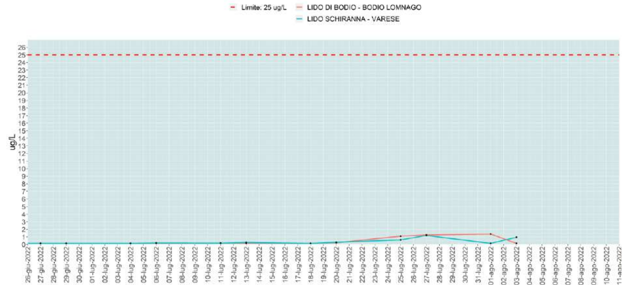
MICROCISTINA
